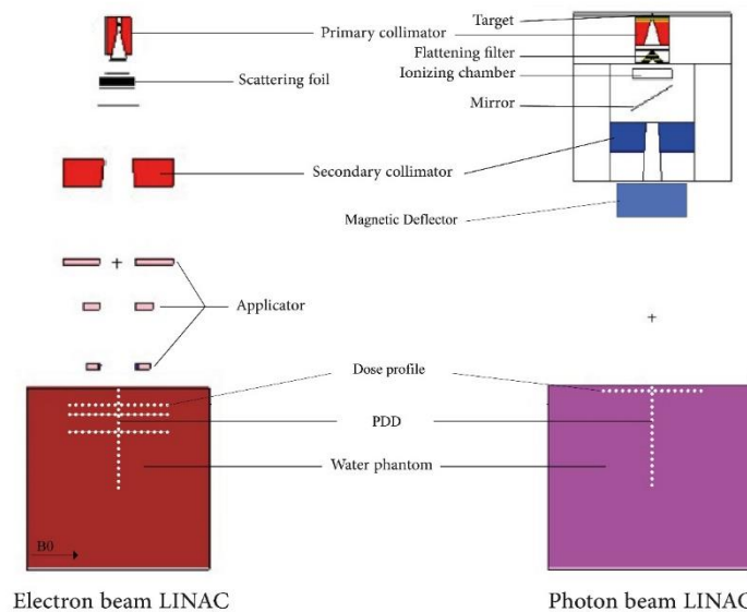
شکل ۱. موقعیت اجزای سر دستگاه LINAC واریان C/D ۲۱۰۰ در دو حالت فوتونی و الکترونی، فانتوم، منحرف‌کننده‌ی مغناطیسی (Magnetic deflector) و شماتیک موقعیت درصد دُز عمقی و پروفایل دُز جذبی در فانتوم
